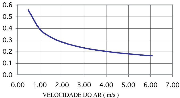
Resistência Térmica ( C/W/4") Código Dissipador: HS 125135
