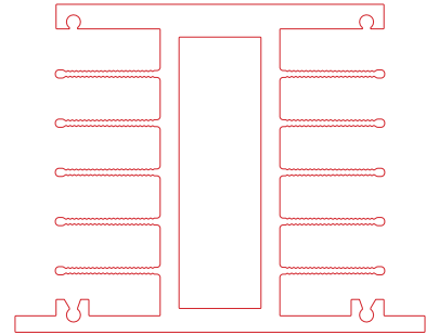
HS 10080
