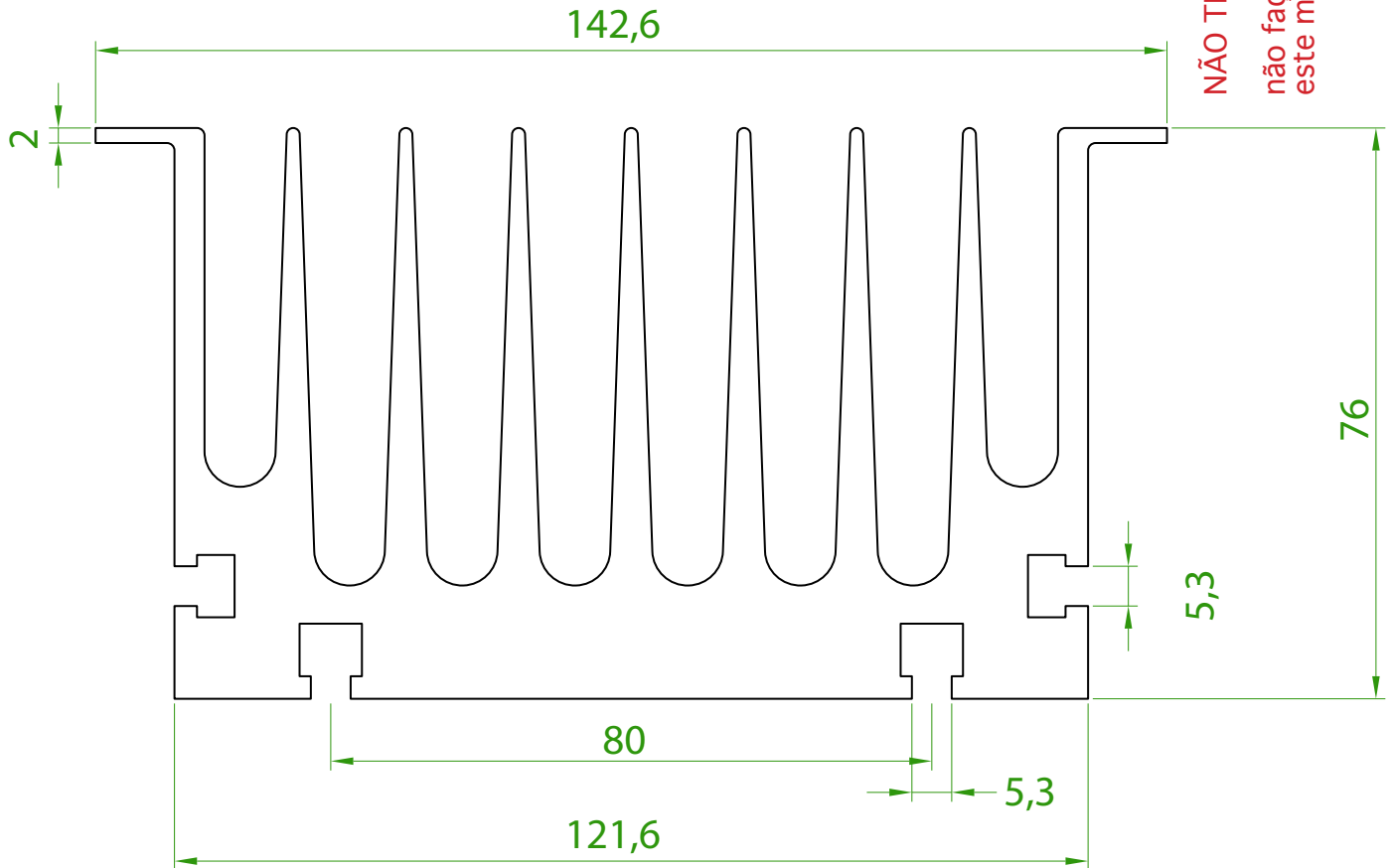
(detalhe)
