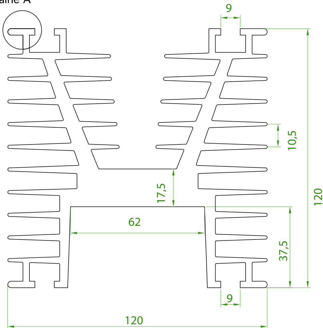
Detalhe A
