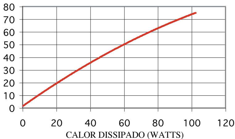
\Delta T C Código Dissipador: HS 125135
